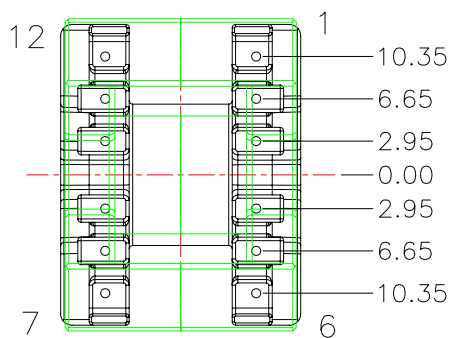
BOTTOM
